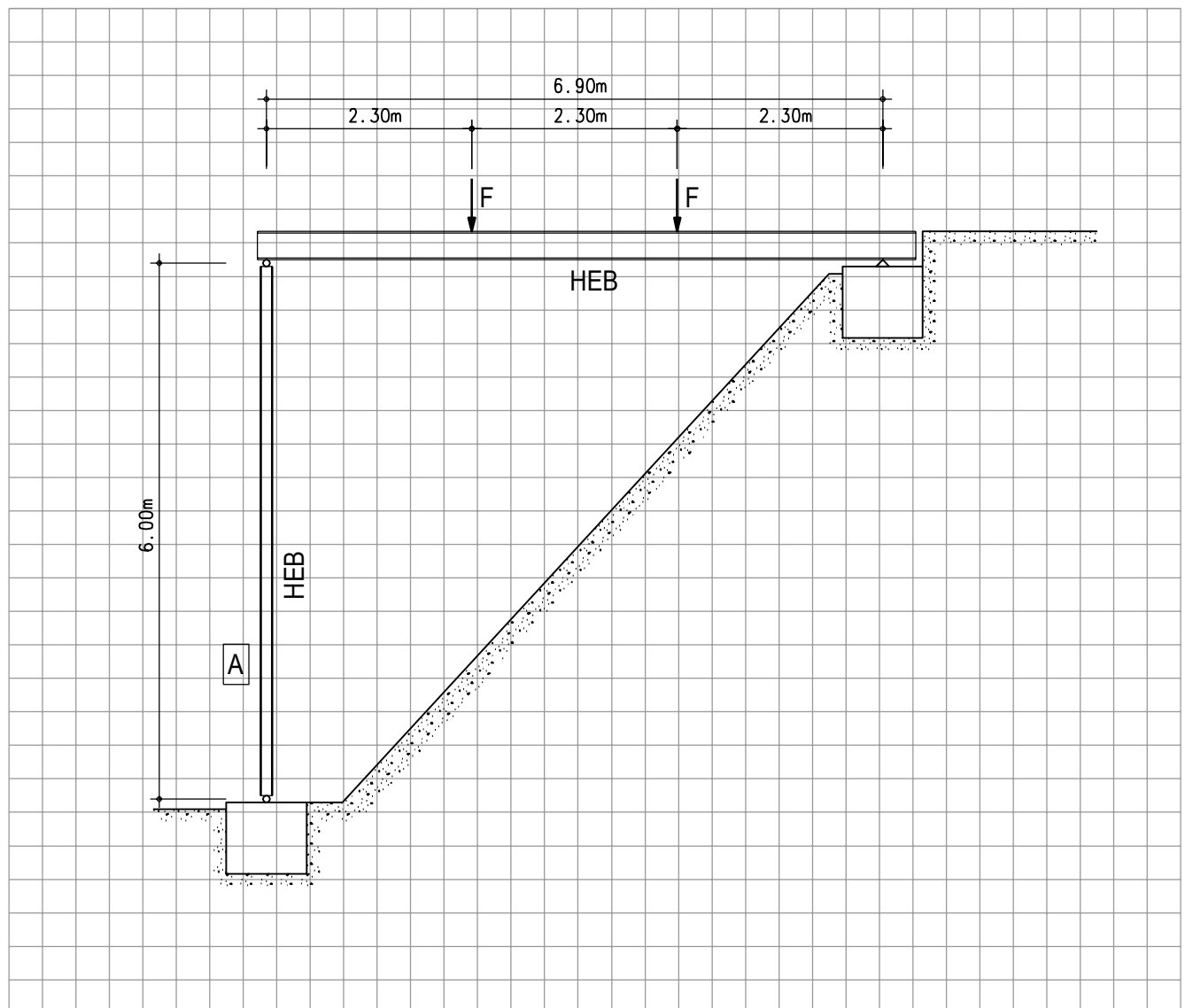
Querschnitt Kranbühne 1:75
