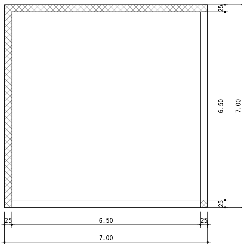
Grundriss 1:75
